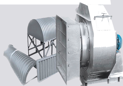
Reposição p/ secador de grãos
