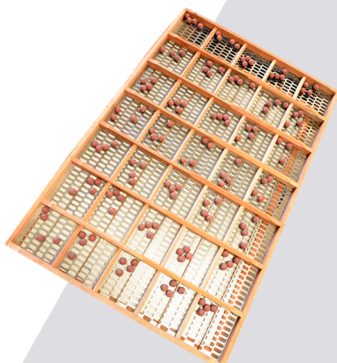
Peneiras para pré-limpeza
